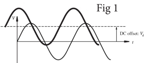
Fig.1) DC-komponent på växelspänningen (oproportionerlig illustrativ figur)
