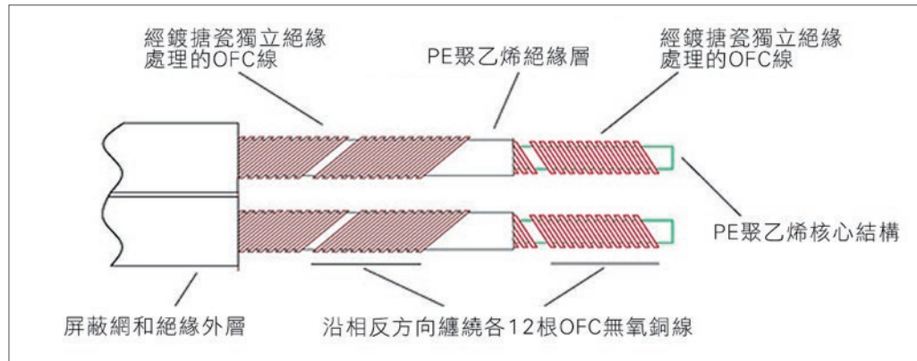
Supra Sword Excalibur 喇叭線內部結構簡化圖。
